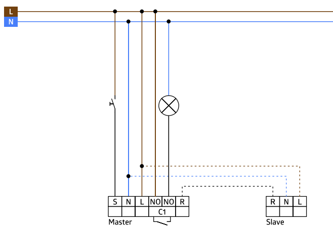
Schakelschema
