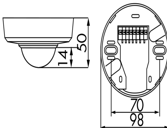
Afmetingen 92305
