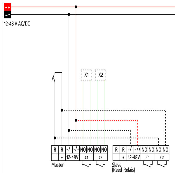
Schakelschema
