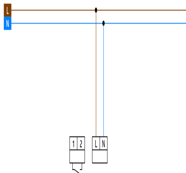
Schakelschema
