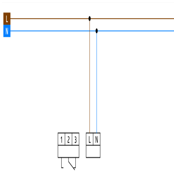
Schakelschema
