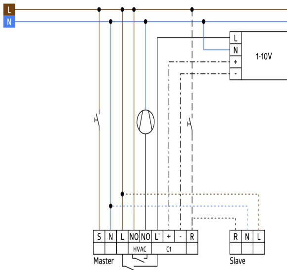
Schakelschema
