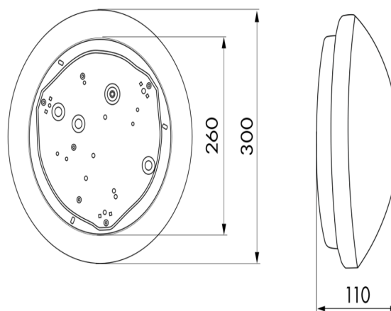
Afmetingen 94445
