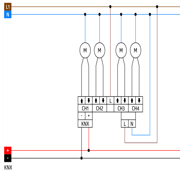
Schakelschema
