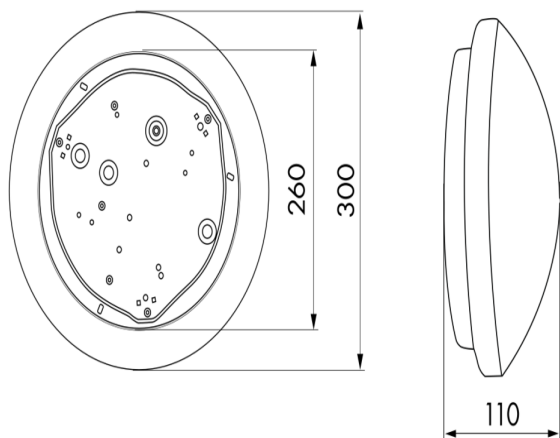
Afmetingen 94451
