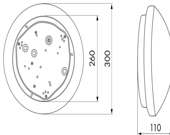
Afmetingen 94446
