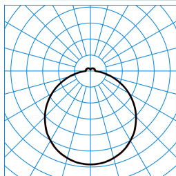
Olisq QWD3 DW 45-840 ETBLE +DMM IP54 IK TX375525
