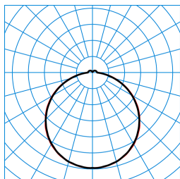
Olisq QWD3 DW 45-840 ETBLE +DMM IP54 IK + Olisq QWD3 ZDR 1/2 03 TX461295
