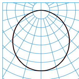
Olisq QWD3 DW 45-840 ETBLE +DMM IP54 IK + Olisq QWD3 ZDR 1/1 03 TX461383
