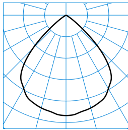
InperiaL G2 C07 BR22 1800-830 01 ■ C0 - C180 TX373312
