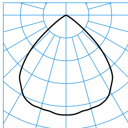
InperiaL G2 C07 BR22 1800-830 01 + DA 01 ■ C0 - C180 TX373309
