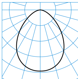
InperiaL G2 C07 BR22 1800-830 01 + DA-M 01 ■ C0 - C180 TX373308
