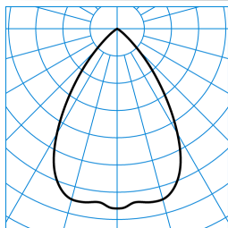
InperiaL G2 C07 BR22 3800-840 ETDD 03 ■ C0 - C180 TX052947
