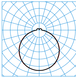
Olisq QWD2 DW 35-840 ETBLE +DMM IK TX376096
