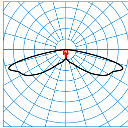
Publisca P1-SB3L/1200-740 2G1S TX047691
