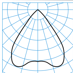
InperiaL G2 C07 HR19 1800-830 03 TX053007 ■ C0 - C180
