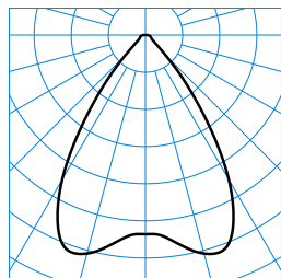
InperiaL G2 C07 HR19 1800-830 03 + ZN-PC TX053012 ■ C0 - C180
