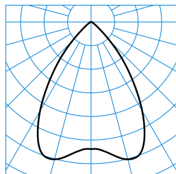
InperiaL G2 C07 HR19 1800-830 03 + RD-PC TX053010 ■ C0 - C180
