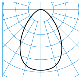
InperiaL G2 C07 HR19 1800-830 03 + DA-M 03 TX053009 ■ C0 - C180
