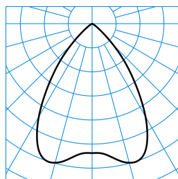
InperiaL G2 C07 HR19 1800-830 03 + DA 03 TX053008 ■ C0 - C180
