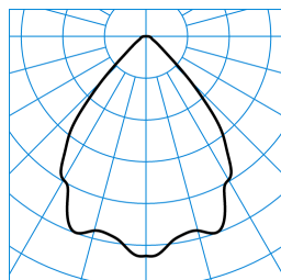
InperlaLP C05 HR22 1800-840 ET EB3 01 + ZN-PC ■ C0 - C180 TX372781
