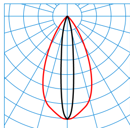
Altigo G2 30 SE6L/1000-830 1G1P + G2 VE IP66 24V DC 120W TX113688
