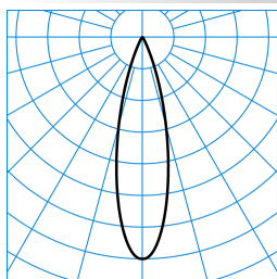
E-Line 7651 LentyP L-MF 40-EC M39 ETDD 01 (150) TX463305
