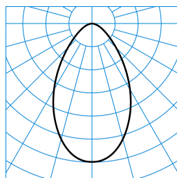
InperiaLP C05 BR22 2700-840 01 + DA-M 03 TX041573 ■ C0 - C180
