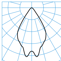
InperiaLP C05 BR22 2700-840 01 + RD-PC TX041574 ■ C0 - C180
