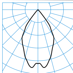
InperiaLP C05 BR22 2700-840 01 TX040953 ■ C0 - C180
