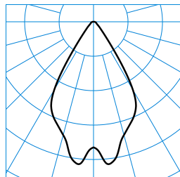
InperiaLP C05 BR22 2700-840 01 + ZN-PC TX041576 ■ C0 - C180
