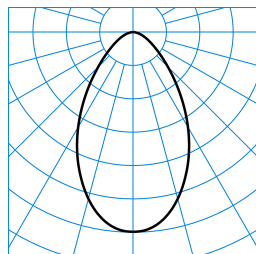
InperiaLP C05 BR22 2700-840 01 + DA-M 01 TX041572 ■ C0 - C180
