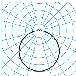
Olisq RWD2 DW 40-830 ET2 IP54 PC + Olisq RWD2 ZDR 1/2 05 TX428260
