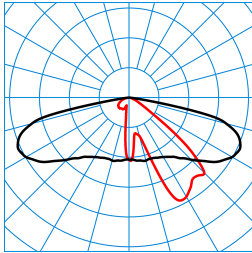
Publisca P1-AB2L-LR/1200-730 2G1S ET (CLO end value) TX300376 ■ C0 - C180 ■ C90 - C270 DIN 5040: A30 UTE: 1,00 G CEN Flux Code: 34 70 96 100 100
