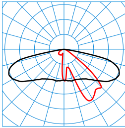
Publisca P1-AB2L-LR/1200-730 2G1S ET (CLO initial value) TX301178 ■ C0 - C180 ■ C90 - C270 DIN 5040: A30 UTE: 1,00 G CEN Flux Code: 34 70 96 100 100
