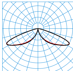
LTX LT-RB6L-LRA/15/18/26-730 4G1 (1800 lm) TX084118
