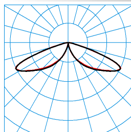
LTX LT-RB6L-LRA/15/18/26-730 4G1 (1500 lm) TX084117
