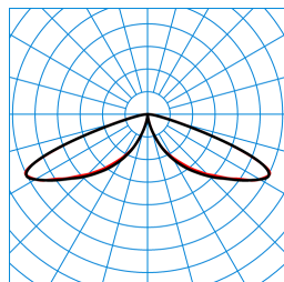
LTX LT-RB6L-LRA/15/18/26-730 4G1 (2600 lm) TX084119
