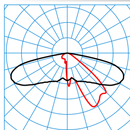
Publisca P2-AB2L-LRA/2200-740 3G1S TX047785 ■ C0 - C180 ■ C90 - C270 DIN 5040: A30 UTE: 1,00 l CEN Flux Code: 34 71 96 100 100
