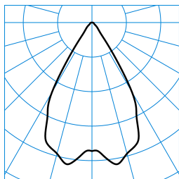
InperiaLP C05 HR22 2700-830 01 + ZN-PC ■ C0 - C180 TX373645
