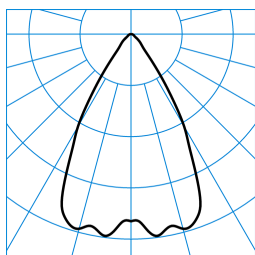
InperiaLP C05 HR22 2700-830 01 + RG-PC ■ C0 - C180 TX373646
