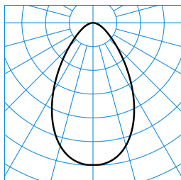
InperiaLP C05 HR22 2700-830 01 + DA-M 03 ■ C0 - C180 TX373648
