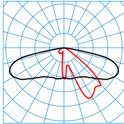
Publisca P1-AB2L-LR/1100-740 2G1S ET (CLO end value) TX300381 ■ C0 - C180 ■ C90 - C270 DIN 5040: A30 UTE: 1,00 G CEN Flux Code: 34 70 96 100 100
