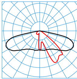
Publisca P1-AB2L-LR/1100-740 2G1S TX047506 ■ C0 - C180 ■ C90 - C270 DIN 5040: A30 UTE: 1,00 G CEN Flux Code: 34 70 96 100 100
