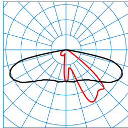
Publisca P1-AB2L-LR/1100-740 2G1S ET (CLO initial value) TX300972 ■ C0 - C180 ■ C90 - C270 DIN 5040: A30 UTE: 1,00 G CEN Flux Code: 34 70 96 100 100
