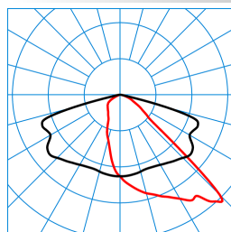
Cuvia 60-AB6L-LR/4200-740 8G1S TX047070
