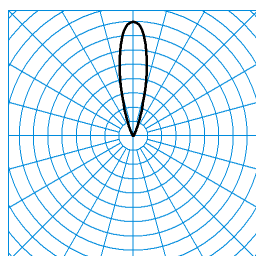
Altigo G2 10 RM3L/350-830 1G1P + G2 VE IP66 24V DC 80W TX113653 ■ C0 - C180
