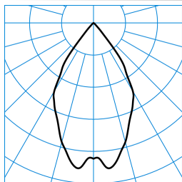
InperlaLP C05 BR19 1800-840 03 TX040942 ■ C0 - C180
