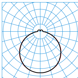
Olisq QWD2 DW 14-40/4/ML-830 IP54 ET (STAGE3) TX425027
