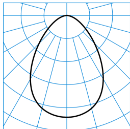
InperlaLP C05 BR22 1800-830 01 + DA-M 03 ■ C0 - C180 TX371306
