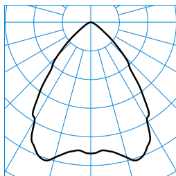
InperiaLP C05 BR22 1800-830 01 + RD-PC TX371307 ■ C0 - C180
