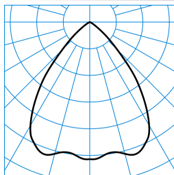
InperiaLP C05 BR22 1800-830 01 TX371302 ■ C0 - C180
