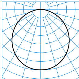
Olisq RWD2 DW 40-840 ETBLE +DMR IP54 PC + Olisq RWD2 ZDR 1/1 01 TX425989
