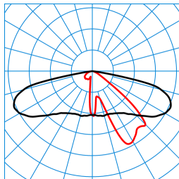
Publisca P1-AB2L-LR/1500-730 2G1S ET (CLO initial value) TX300442 ■ C0 - C180 ■ C90 - C270 DIN 5040: A30 UTE: 1,00 G CEN Flux Code: 34 70 96 100 100
