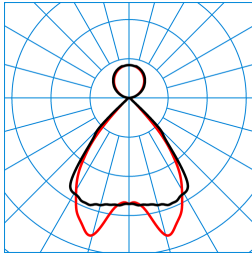
SFlow H3-L MRX LED6400-840 LLWM 01 TX053176
