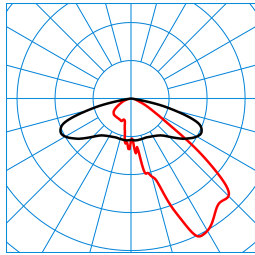
Publisca P1-AB2L/2900-730 4G1S TX047488
