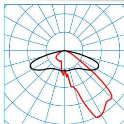
Publisca P2-AB2L-LRA/2900-730 4G1S TX047790 ■ C0 - C180 ■ C90 - C270 DIN 5040: A30 UTE: 1,00 G CEN Flux Code: 35 73 97 100 100
