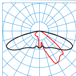
Publisca P1-AB2L-LRA/4600-730 6G1S TX047572 ■ C0 - C180 ■ C90 - C270 DIN 5040: A30 UTE: 1,00 G CEN Flux Code: 35 74 97 100 100
