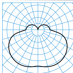
PolaroniQ WD1D LED1000-840 ET TX370237
