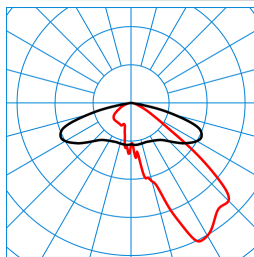
Publisca P2-AB2L-LR/2900-730 4G1S TX047753 DIN 5040: A30 UTE: 1,00 G CEN Flux Code: 35 73 97 100 100 ■ C0 - C180 ■ C90 - C270
