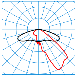
Publisca P2-AB2L-LRA/3200-740 4G1S ET (CLO end value) TX300322 ■ C0 - C180 ■ C90 - C270 DIN 5040: A30 UTE: 1,00 G CEN Flux Code: 35 73 97 100 100
