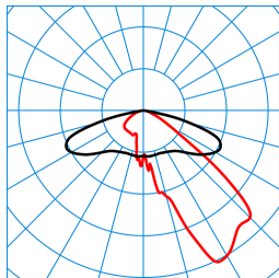
Publisca P2-AB2L-LRA/3200-740 4G1S ET (CLO initial value) TX300546 ■ C0 - C180 ■ C90 - C270 DIN 5040: A30 UTE: 1,00 G CEN Flux Code: 35 73 97 100 100
