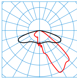
Publisca P2-AB2L-LRA/3200-740 4G1S TX047793 ■ C0 - C180 ■ C90 - C270 DIN 5040: A30 UTE: 1,00 G CEN Flux Code: 35 73 97 100 100
