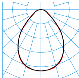
ArimoFit G2 M59 PW19 63-840 ETDD + ArimoFit G2 Sky M59-TS ZER TX426837
