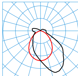
TugraHE Act 15 PAW 60-840 ETDD8 01 (ACTDCW) TX302961 ■ C0 - C180 ■ C90 - C270 DIN 5040: B40 UTE: 0,87 E + 0,13 T CEN Flux Code: 48 79 93 87 100 7 25 60 13
