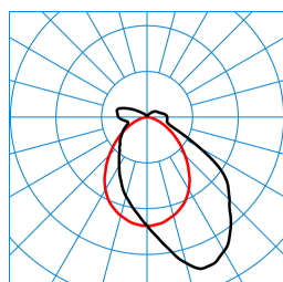
TugraHE Act 15 PAW 60-840 ETDD8 01 (ACTDSU) TX302747 ■ C0 - C180 ■ C90 - C270 DIN 5040: B40 UTE: 0,87 E + 0,13 T CEN Flux Code: 48 79 93 87 100 7 25 60 13
