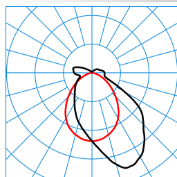
TugraHE Act 15 PAW 60-840 ETDD8 01 (ACTDWW) TX302914 ■ C0 - C180 ■ C90 - C270 DIN 5040: B40 UTE: 0,87 E + 0,13 T CEN Flux Code: 48 79 93 87 100 7 25 60 13
