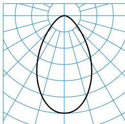
InperiaLP C05 BR19 1800-840 01 + DA-M 01 TX370771 ■ C0 - C180
