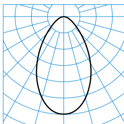
InperiaLP C05 BR19 1800-840 01 + DA-M 03 TX370772 ■ C0 - C180
