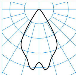
InperiaLP C05 BR19 1800-840 01 + ZN-PC TX370775 ■ C0 - C180
