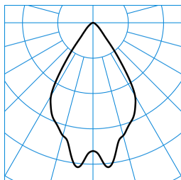
InperiaLP C05 BR19 1800-840 01 + RD-PC TX370773 ■ C0 - C180
