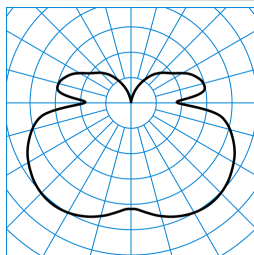
PolaroniQ W2D LED2000-830 ETDD TX040709
