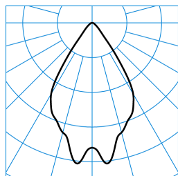
InperiaLP C05 BR22 2700-830 01 + RG-PC ■ C0 - C180 TX041561
