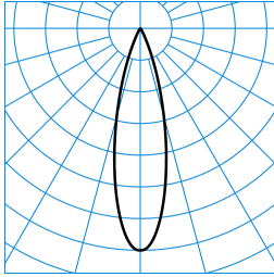
E-Line 7651 Lentyp L-MF 20-BF M54 ET 05 (225) TX463290
