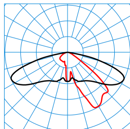
Publisca P2-AB2L-LR/3800-740 6G1S ET (CLO initial value) TX301197 ■ C0 - C180 ■ C90 - C270 DIN 5040: A30 UTE: 1,00 G CEN Flux Code: 35 74 97 100 100
