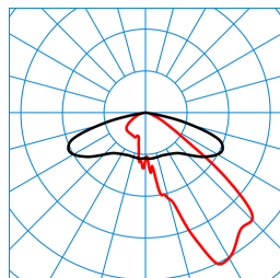
Publisca P1-AB2L-LRA/2900-740 4G1S ET (CLO initial value) TX300405 ■ C0 - C180 ■ C90 - C270 DIN 5040: A30 UTE: 1,00 G CEN Flux Code: 35 73 97 100 100
