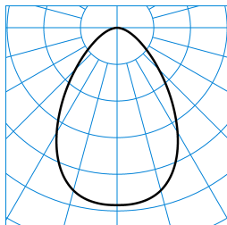
InperiaL G2 C07 BR22 3800-830 01 + DA-M 01 ■ C0 - C180 TX373091
