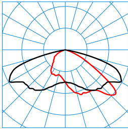
LIQ 70N-AB7L-LRA/10000-727 12G1 ETDD(CLO end value) TX278165
