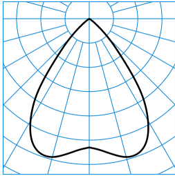
InperiaL G2 C07 BR19 1800-840 01 ■ C0 - C180 TX372402
