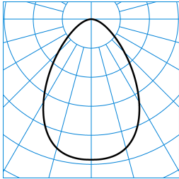
InperiaL G2 C07 BR19 1800-840 01 + DA-M 01 ■ C0 - C180 TX372404
