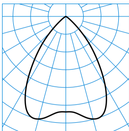
InperiaL G2 C07 BR19 1800-840 01 + DA 01 ■ C0 - C180 TX372403
