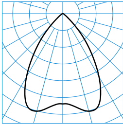
InperiaL G2 C07 BR19 1800-840 01 + RD-PC ■ C0 - C180 TX372405
